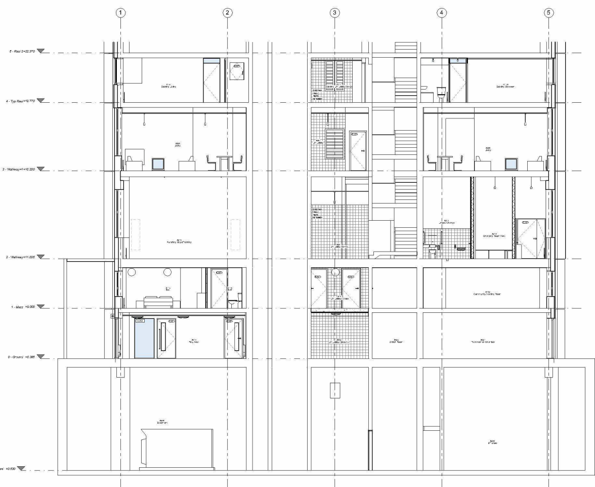
Section B 1 : 50
